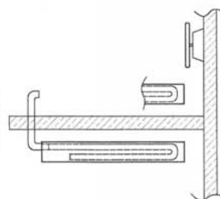
Leitungsverlauf Beschickung
