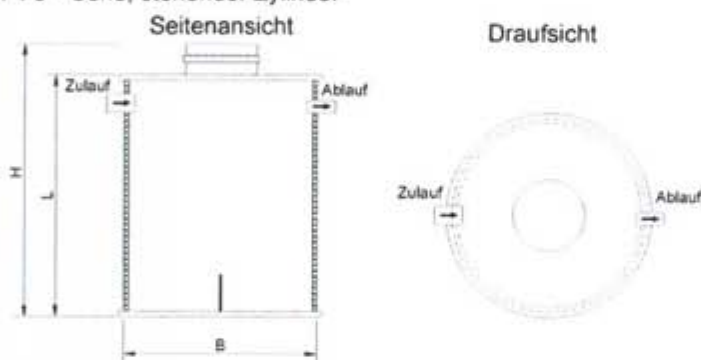
Behälter C PE - Behälter TO - Serie, stehender Zylinder
